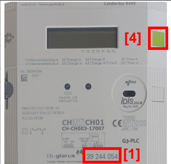
Elektronischer Zähler, Landis+Gyr E450s4 Smart Meter
